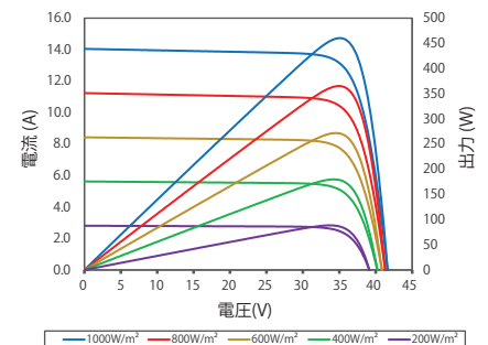
IV 特性データ
